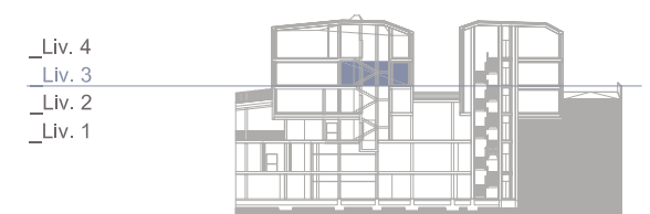
SEZIONE BB
